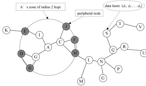
Fig. 1. A MANET
