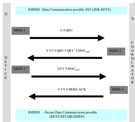
Fig. 5. SKKE protocol
